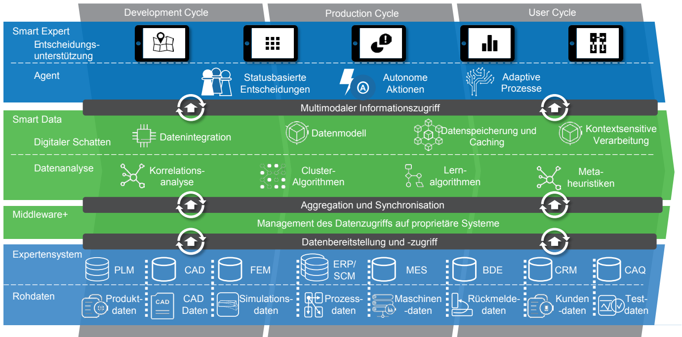
Infrastruktur des Internet of Production
